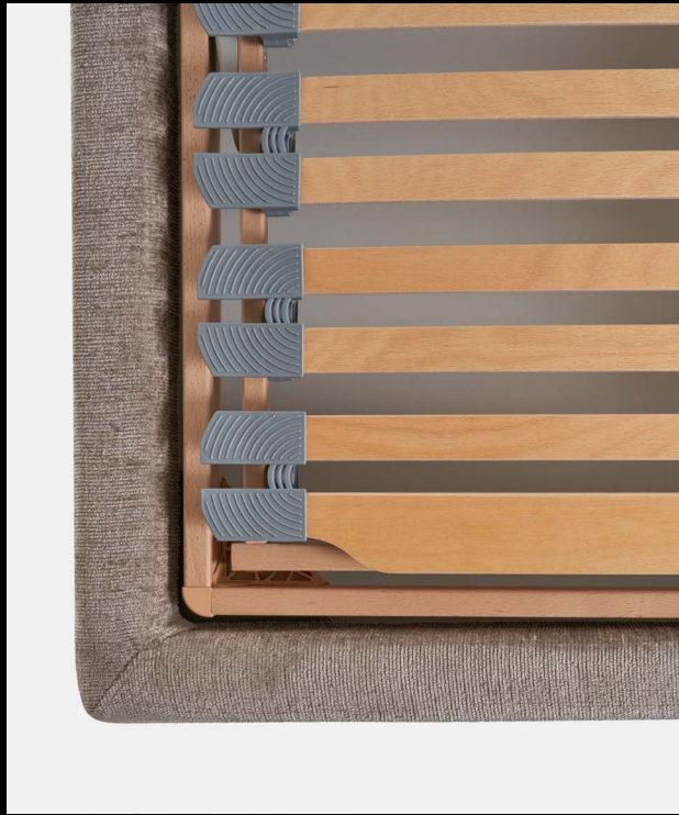
SPESSORE SOMMIER EVOLUZIONE Thickness of the Evolution bed base Épaisseur du sommier Évolution
